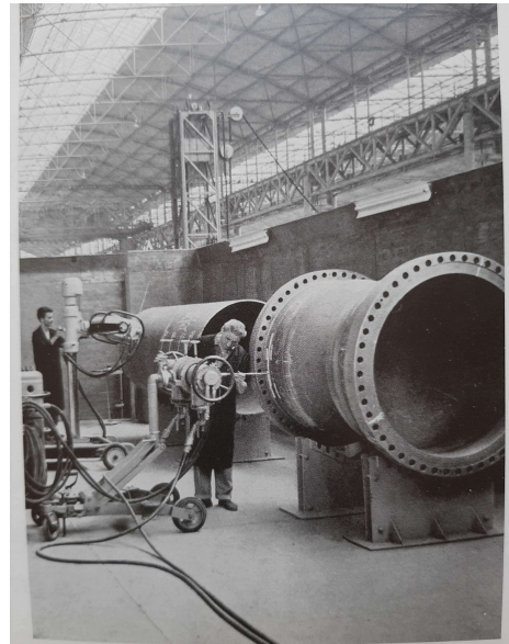
Azienda Bonaldi. Apparecchiatura per radiografie alle saldature di precisione
